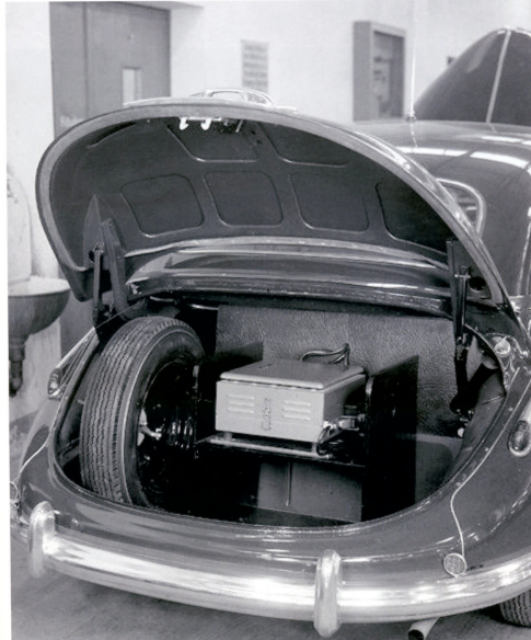
Lorenz SEM 7 Geräteblock - Schaubild (linke Seite)
