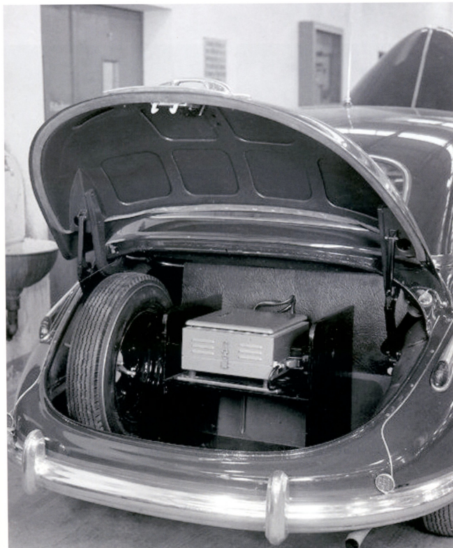
Lorenz SEM 7 Geräteblock - Schaubild (linke Seite)
