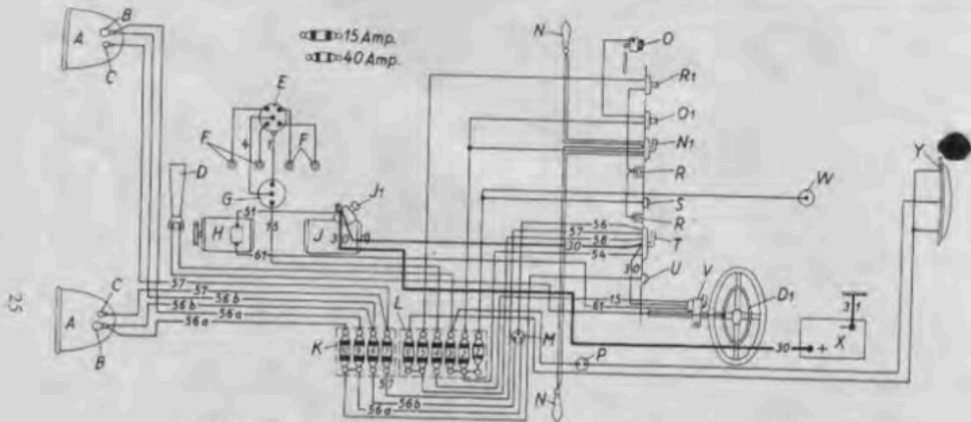
Bild 13. Schaltung der elektrischen Einrichtungen (Batterie-Kontrolllampe am Sicherungsschloß)
